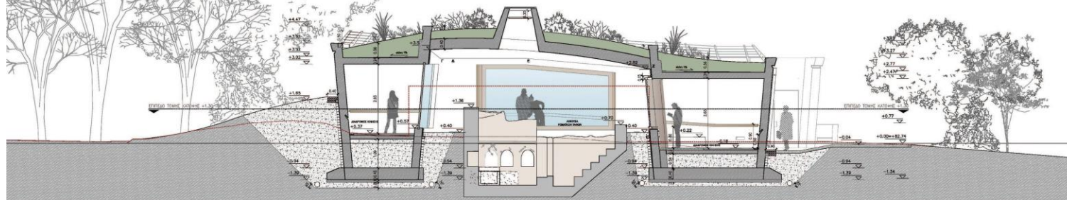
ΤΟΜΗ Γ-Γ
